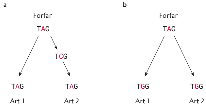
Figur 16. Flere mutationer i samme baseposition.
