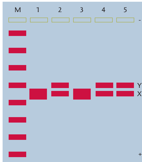
Figur 39. Kønsbestemmelse via amelogenin-genet.
